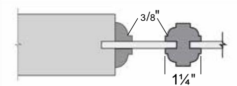
TDL Ovolo Bead
